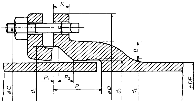
부표 1-1 - 메커니컬 조인트관의 소켓
