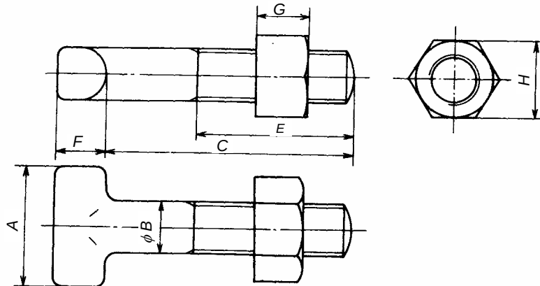
부표 1-3 - 메커니컬 조인트용 볼트·너트
