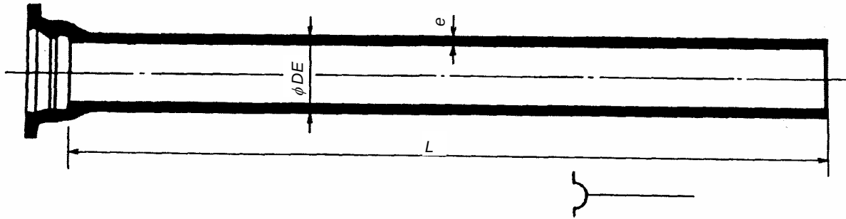
부표 1-8 - 메커니컬 조인트 4종관
