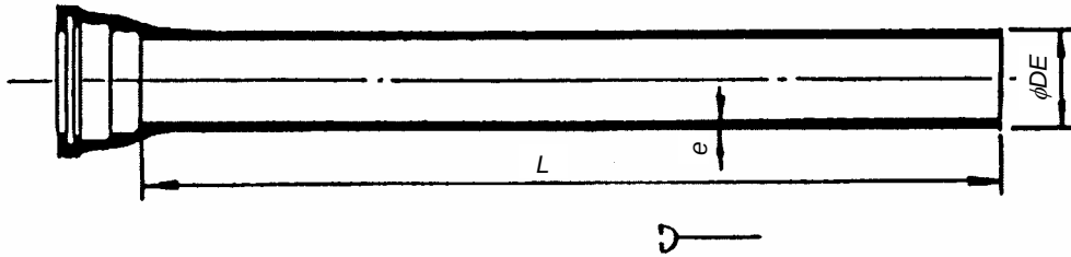
부표 3-5 - 타이튼 조인트 3종관
