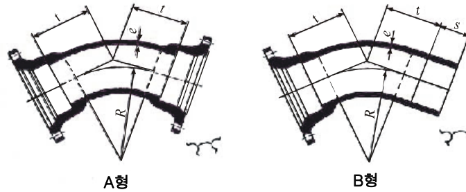
부표 1-8 — 메커니컬 조인트, 45도 소켓 곡관
