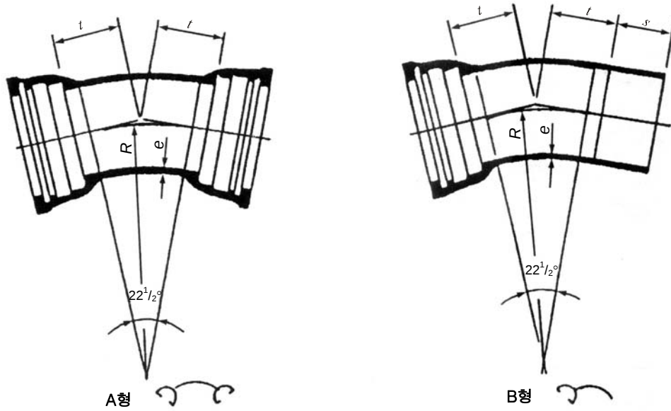
부표 3-6 - 타이튼 조인트, 22\frac{1}{2}^\circ 도 소켓 곡관
