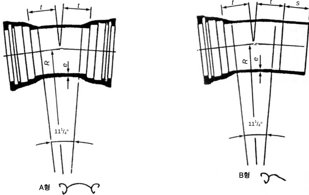
부표 3-7 - 타이튼 조인트, 11\frac{1}{4} 도 소켓 곡관
