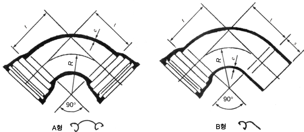
부표 3-4 - 타이튼 조인트, 90도 소켓 곡관
