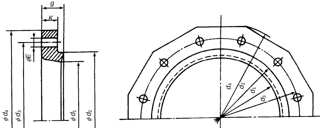
부표 1-2 - 메커니컬 조인트용 압륜
