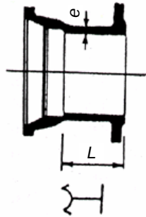
부표 2-5 - KP 메커니컬 조인트, 플랜지 소켓관
