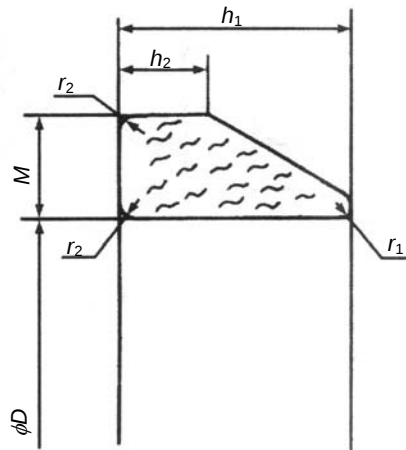
부표 1-4 - 메커니컬 조인트용 고무링
