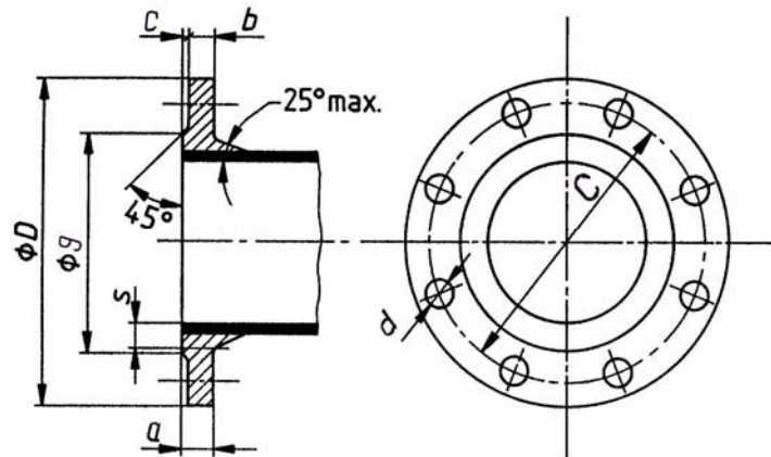
부표 4-1 - 플랜지(PN 10)
