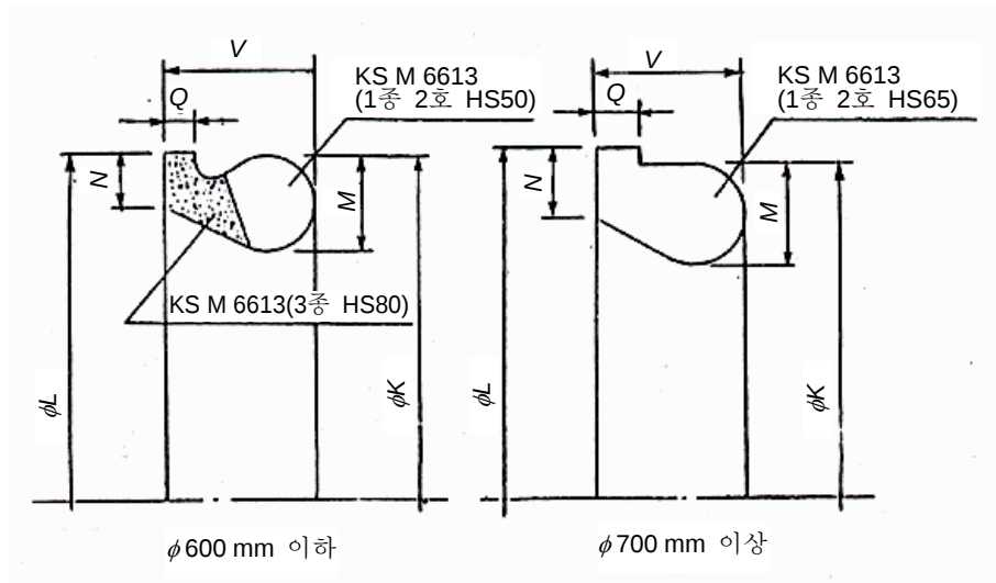
부표 3-2 - 타이튼 조인트용 고무링
