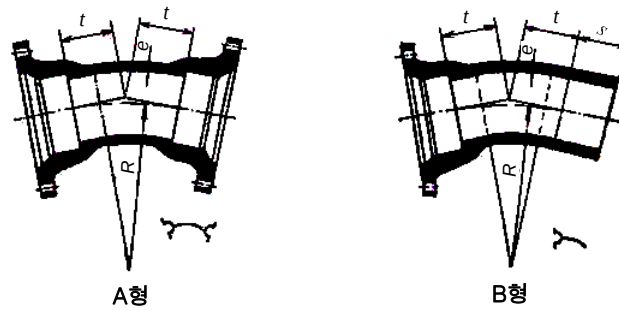
부표 1-9 - 메커니컬 조인트, 22 1/2도 소켓 곡관
