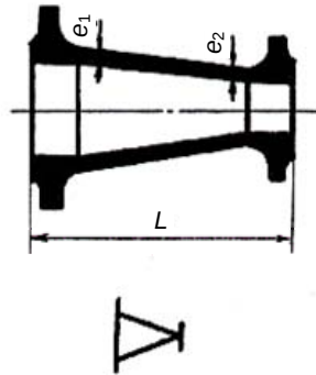
부표 4-4 — 플랜지 편락관
