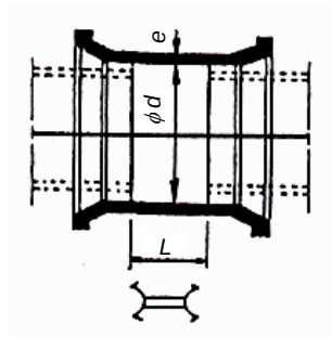
부표 2-6 - KP 메커니컬 조인트, 이음관
