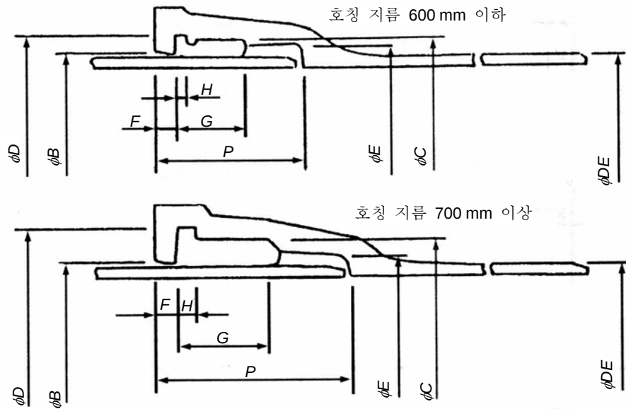
부표 3-1 - 타이튼 조인트관의 소켓
