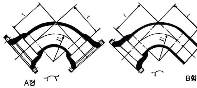
부표 1-7 — 메커니컬 조인트, 90도 소켓 곡관
