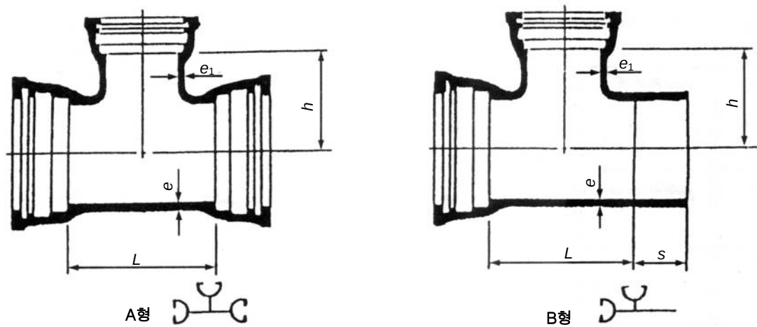
부표 3-9 - 타이튼 조인트, 소켓 T형관
