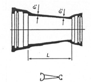
부표 3-10 - 타이튼 조인트, 소켓 편락관
