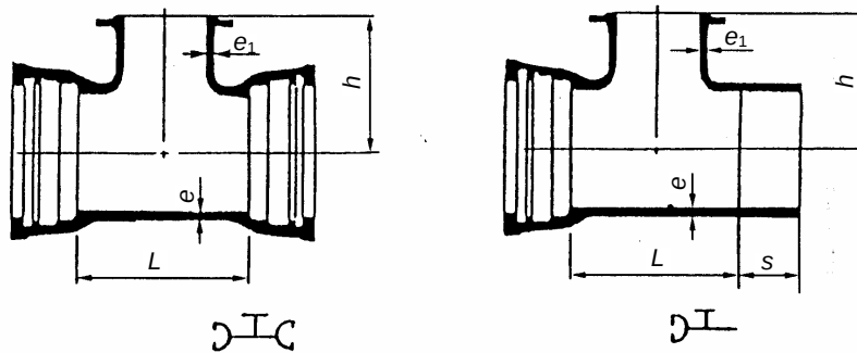
부표 3-8 - 타이튼 조인트, 소켓 플랜지 T형관
