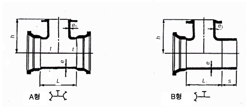
부표 2-11 — KP 메커니컬 조인트, 소켓 플랜지 T형관
