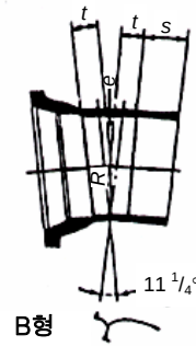
부표 2-10 — KP 메커니컬 조인트, 11\frac{1}{4} 도 소켓 곡관
