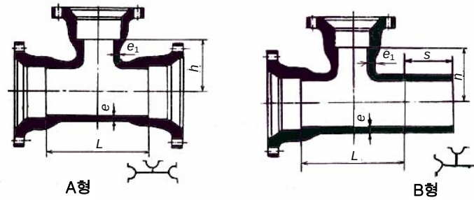
부표 1-12 — 메커니컬 조인트, 소켓 T형관
