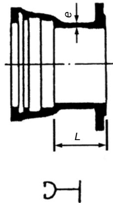
부표 3-3 — 타이튼 조인트, 플랜지 소켓관
