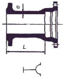
부표 1-5 — 메커니컬 조인트 플랜지 소켓관
