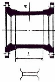
부표 1-6 — 메커니컬 조인트 이음관
