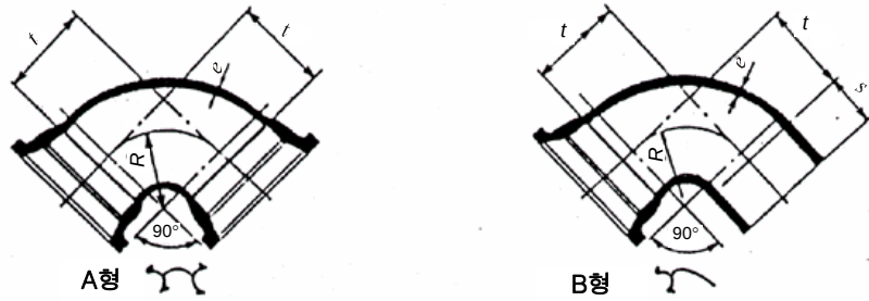
부표 2-7 - KP 메커니컬 조인트 90도 소켓 곡관
