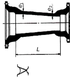
부표 1-13 - 메커니컬 조인트, 소켓 편락관
