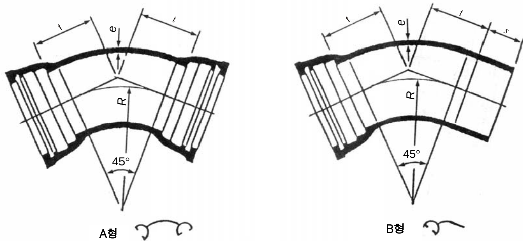
부표 3-5 - 타이튼 조인트, 45도 소켓 곡관
