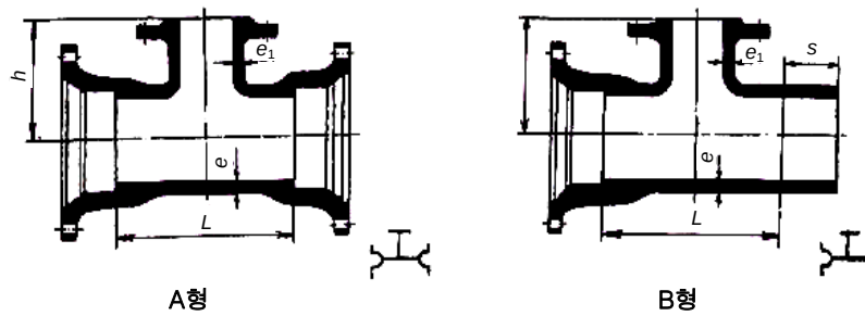
부표 1-11 — 메커니컬 조인트 소켓 플랜지 T형관
