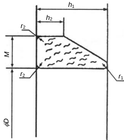
부표 2-4 — KP 메커니컬 조인트용 고무링
