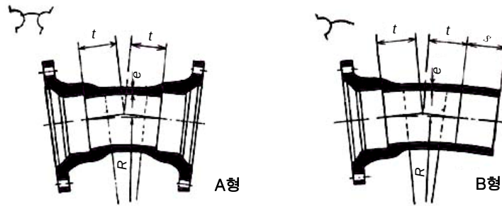
부표 1-10 — 메커니컬 조인트, 11 1/4도 소켓 곡관
