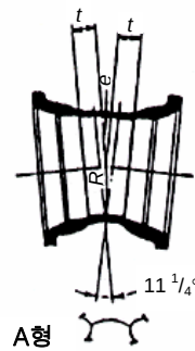
부표 2-10 — KP 메커니컬 조인트, 11\frac{1}{4} 도 소켓 곡관
