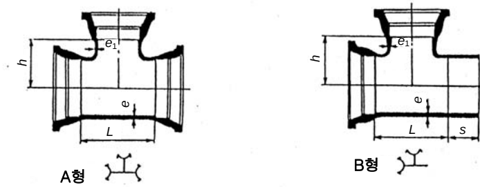
부표 2-12 — KP 메커니컬 조인트, 소켓 T형관
