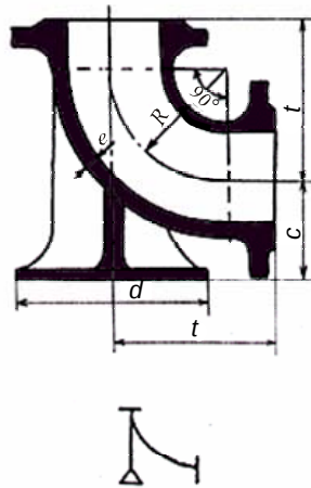
부표 4-7 — 플랜지 소화전 곡관
