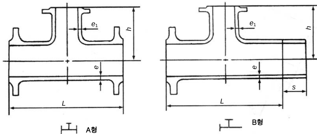
부표 4-9 - 플랜지 T형관
