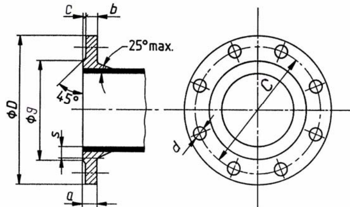
부표 4-2 — 플랜지(PN 16)
