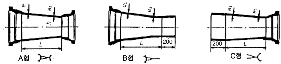
부표 2-13 - KP 메커니컬 조인트, 소켓 편락관
