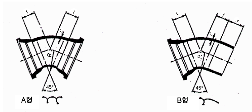
부표 2-8 - KP 메커니컬 조인트 45도 소켓 곡관
