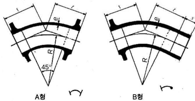
부표 4-8 — 45도 플랜지 곡관
